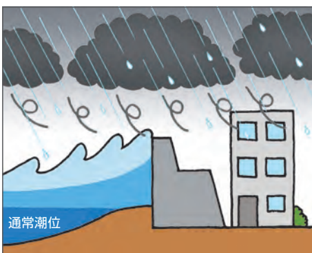
大気圧の低下に伴う「吸い上げ効果」と、陸に向かって吹く強風による「吹き寄せ効果」によってさらに海水面が上がる。
