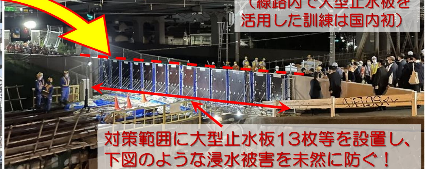
増水時の越水防止対策 (止水壁完成状況)
